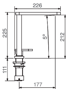
Bica levantada
